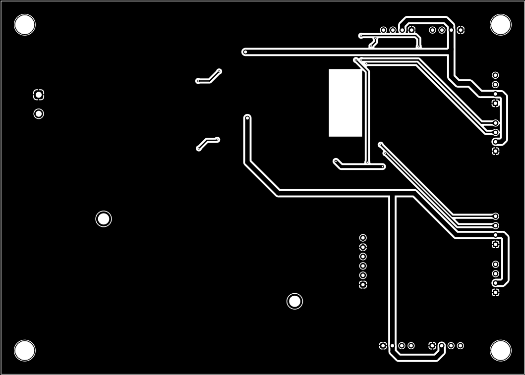
Нижний проводящий рисунок (1:1)
