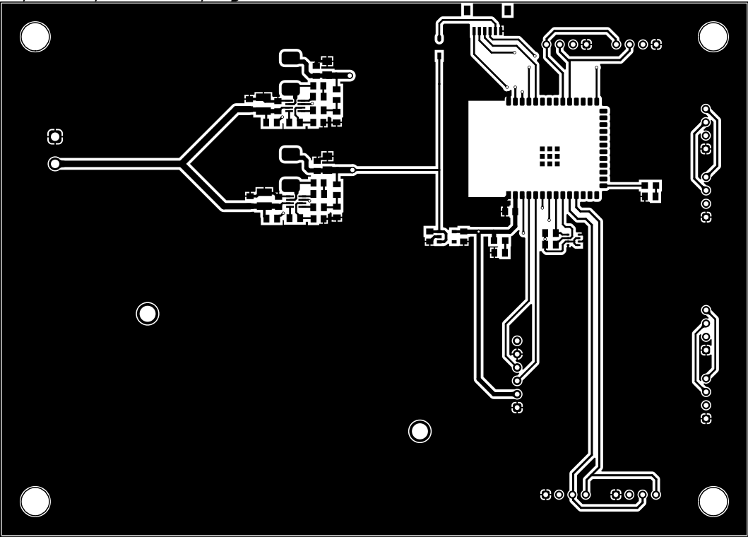
Верхний проводящий рисунок (1:1)
