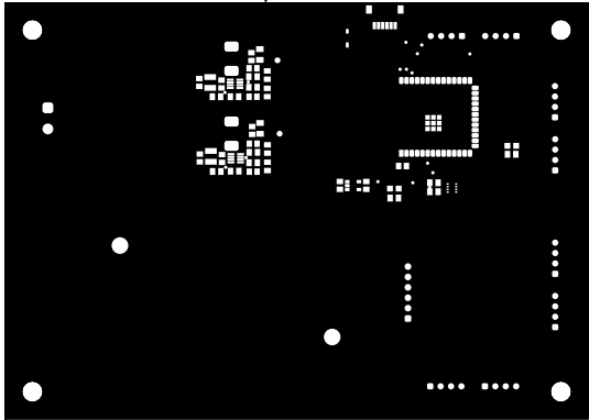
Масочный слой верхнего слоя (1:2)
